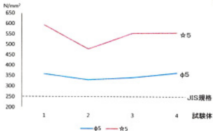
溶接部引張試験 (JIS規格250N/mm 2 以上)
