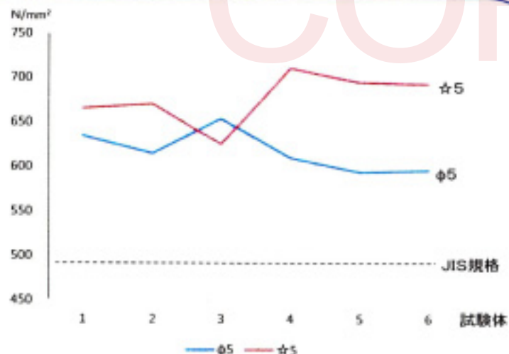
材料引張試験 (JIS規格490N/mm 2 以上)
